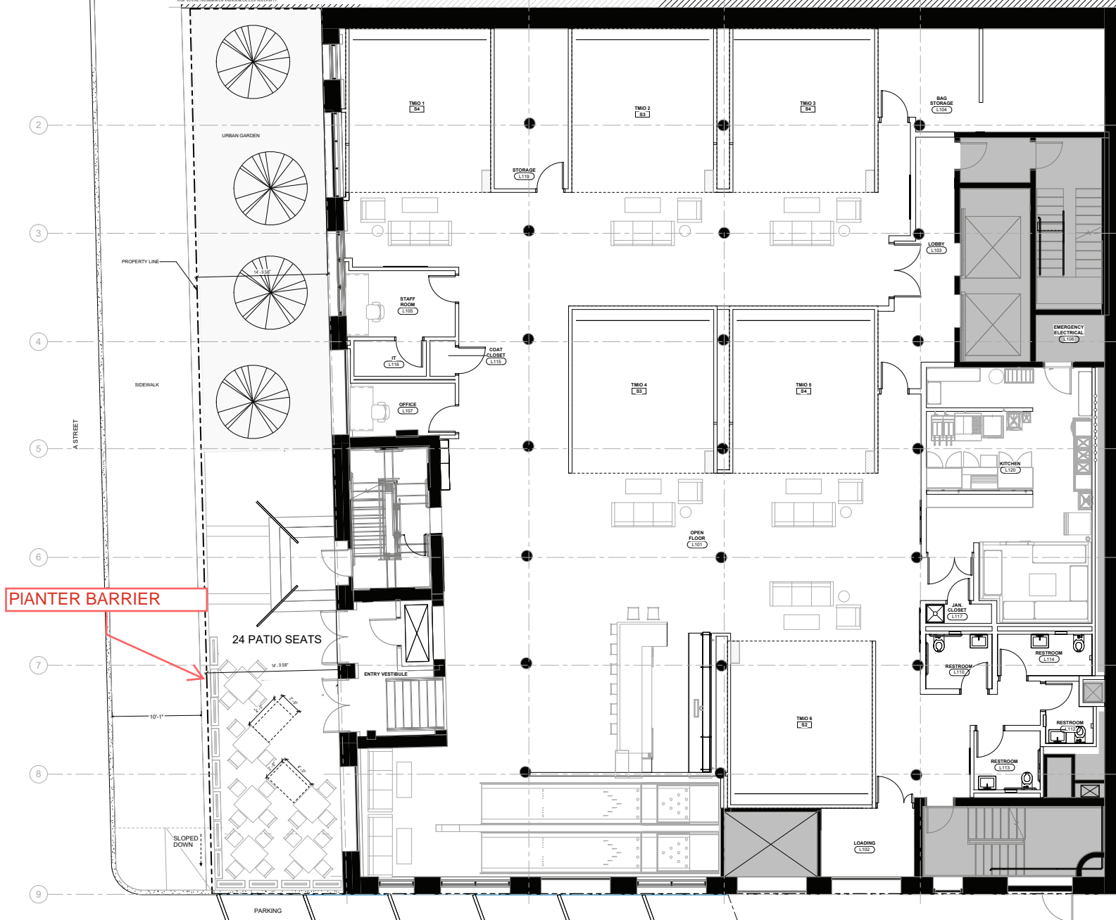
1 PREMISE USE PLAN SCALE: 1/4" = 1'-0"
